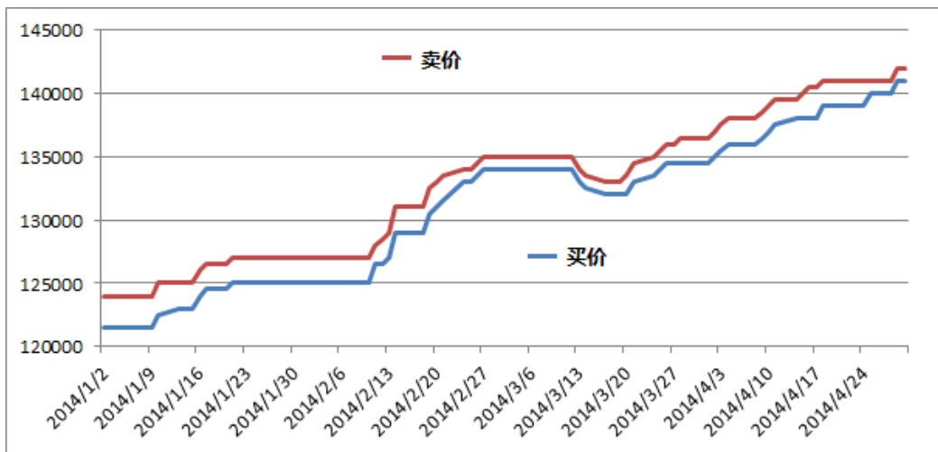
图 1:2014 年 1-4 月国内市场精铋价格走势（元/吨）
